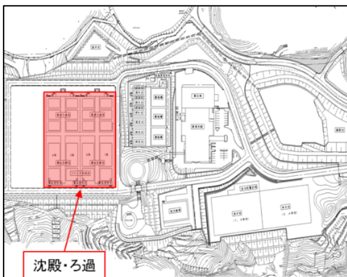
(すりかみ浄水場内配置図)
