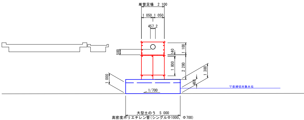
A-A'断面図 S=1:100 (A1) S=1:200 (A3)
