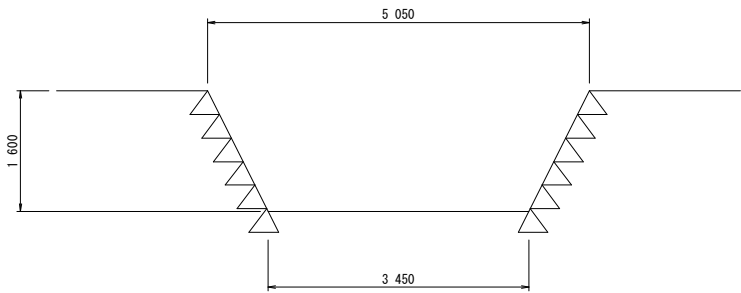
河川断面図 S=1:50 (A1) S=1:100 (A3)
