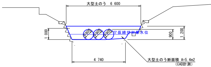
詳細断面図 S=1:20 (A1) S=1:40 (A3)
