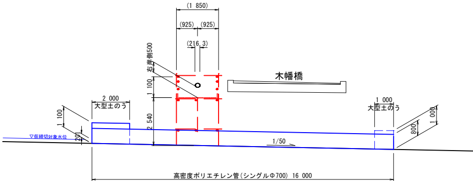
A-A'断面図 S=1:100 (A1) S=1:200 (A3)
