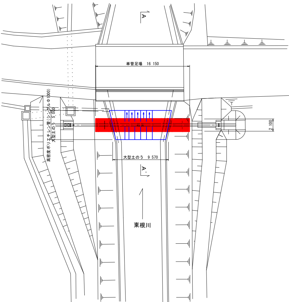
平面図 S=1:200 (A1) S=1:400 (A3)
