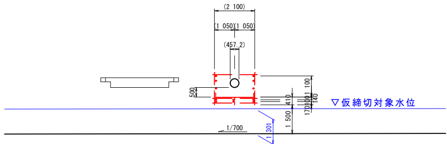
A-A'断面図 S=1:100 (A1) S=1:200 (A3)
