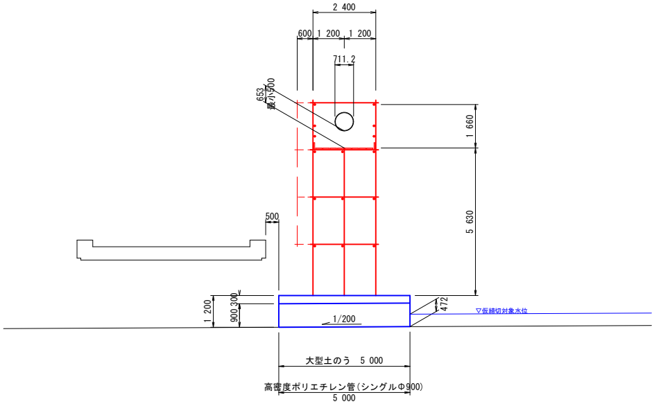
A-A'断面図 S=1:100 (A1) S=1:200 (A3)
