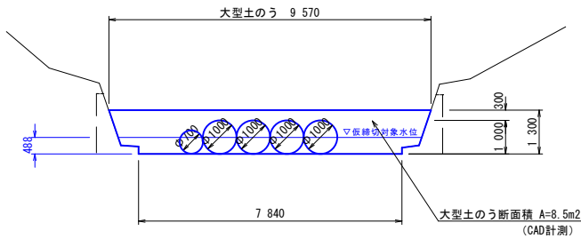
仮締切断面図 S=1:100 (A1) S=1:200 (A3)
