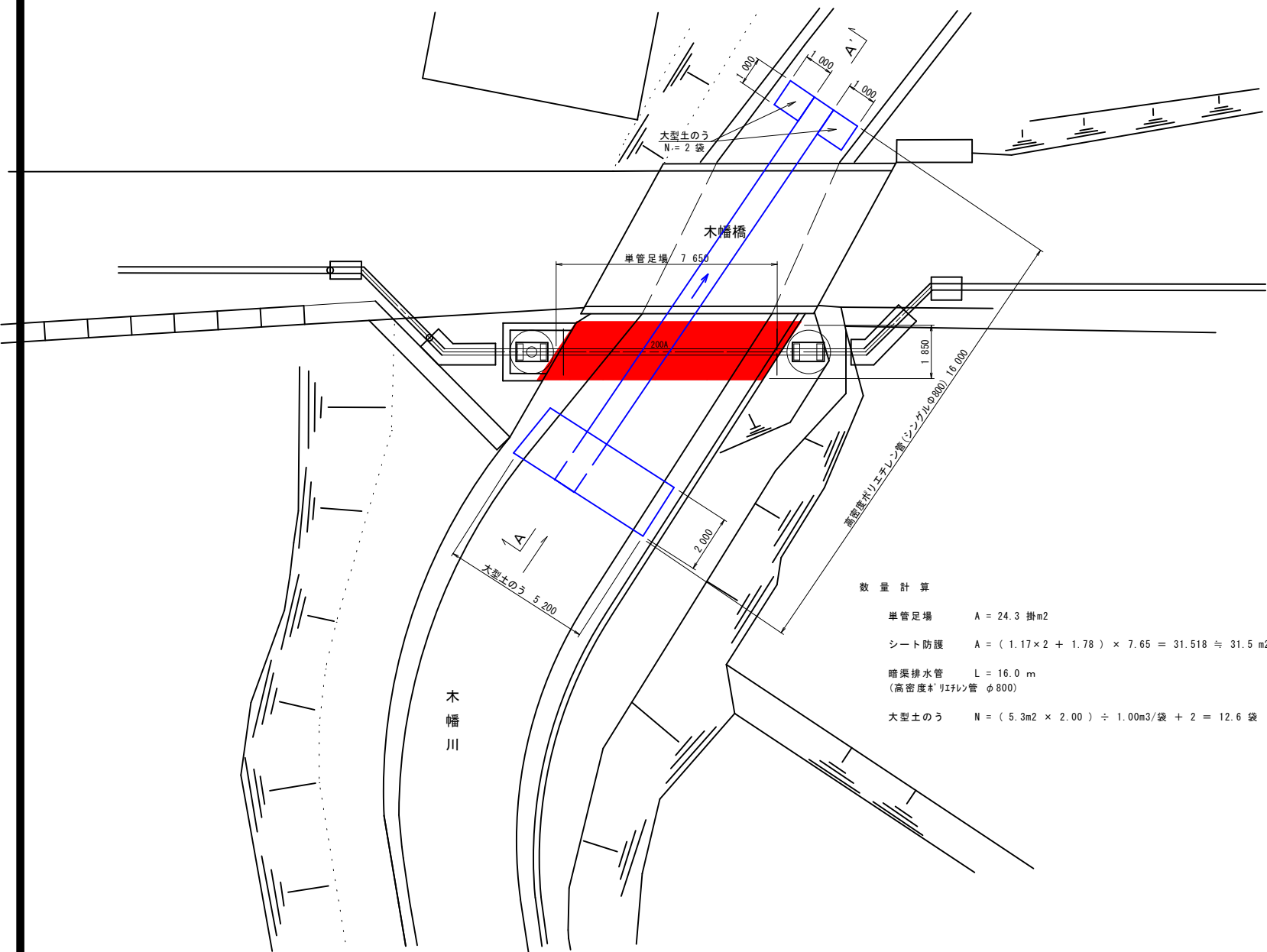
平面図 S=1:100 (A1) S=1:200 (A3)
