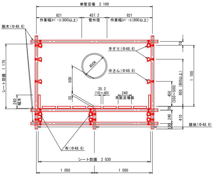
詳細断面図 S=1:20 (A1) S=1:40 (A3)
