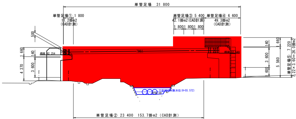
側面図 S=1:200 (A1) S=1:400 (A3)
