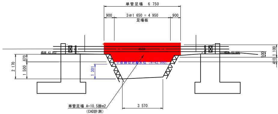
側面図 S=1:100 (A1) S=1:200 (A3)
