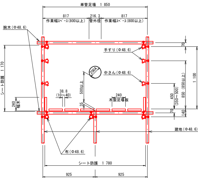
詳細断面図 S=1:20 (A1) S=1:40 (A3)
