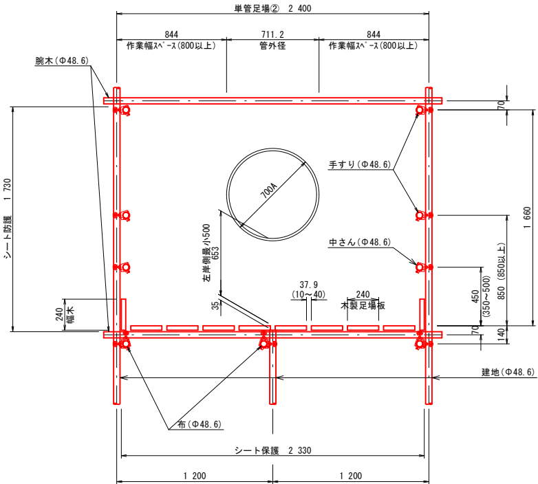
詳細断面図 S=1:20 (A1) S=1:40 (A3)
